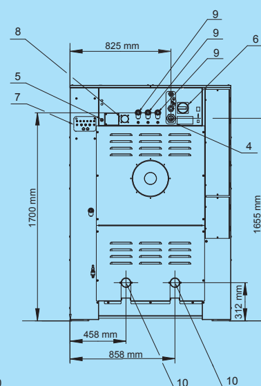
Lado traseiro
